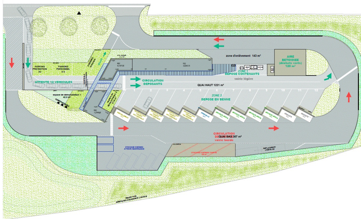
Plan de masse de la déchetterie
